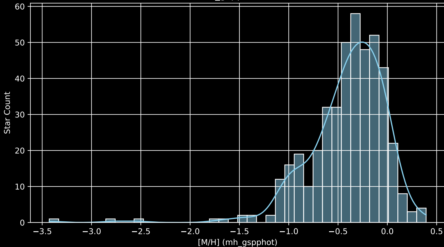
GALAH DR4 Field: [6595] [M/H] (mh_gspphot) (n= 440)
