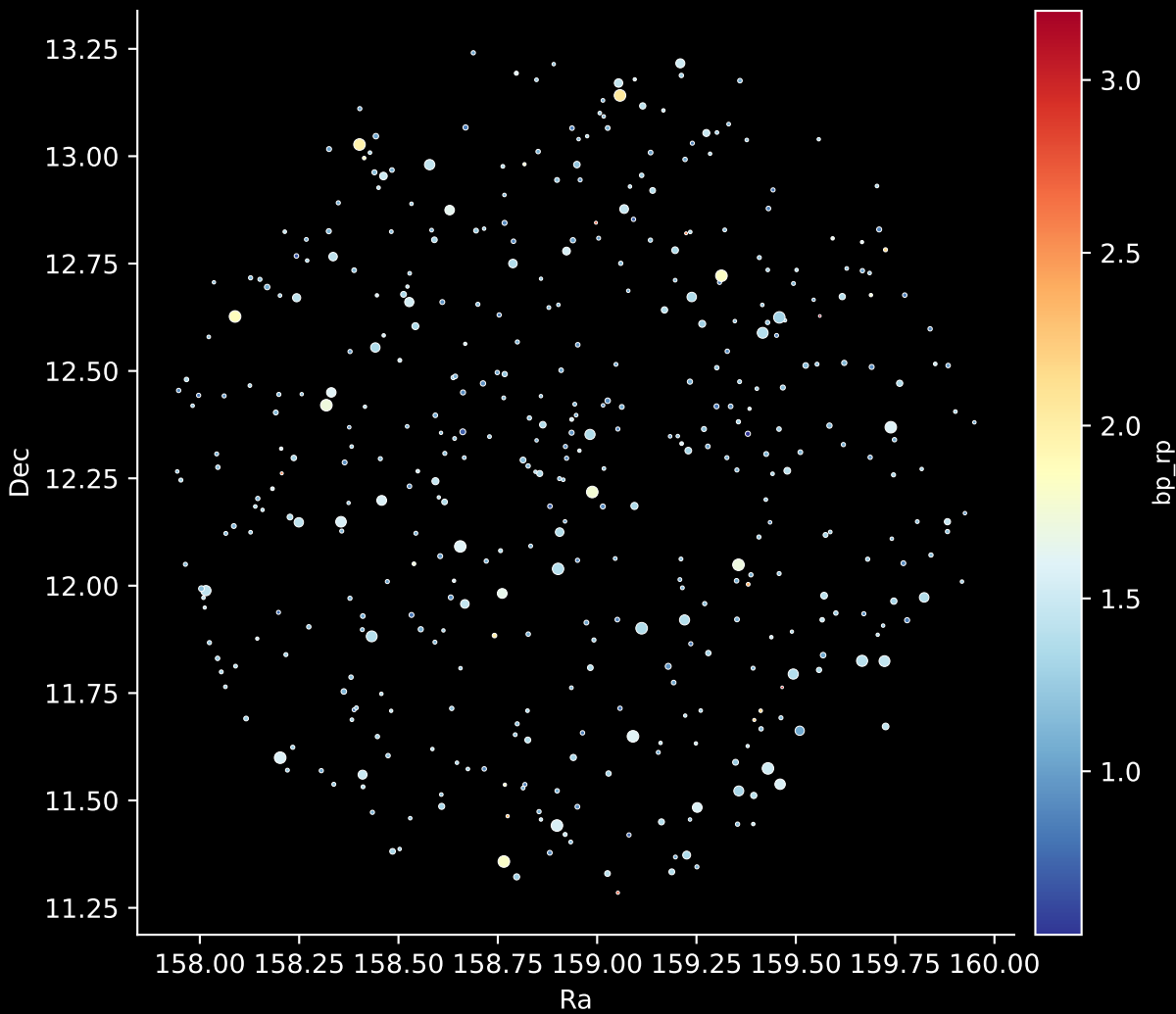
GALAH DR4 Field: [6595] Stars: 441
